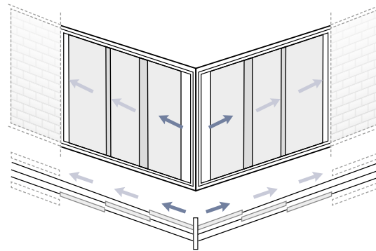
2 x 3 vantaux
