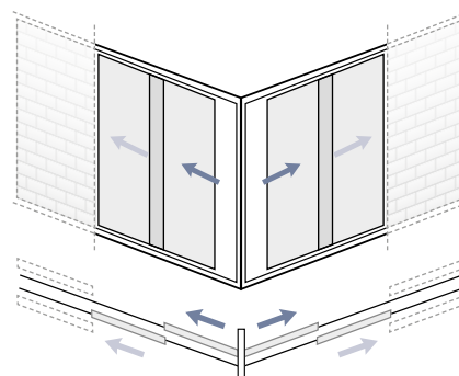
2 x 2 vantaux
