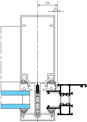
coupe ouverture extérieure
